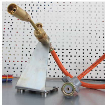
Eingasbrenner
